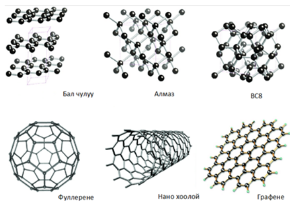
Зураг 1. Нүүрстөрөгчийн аллотропууд
