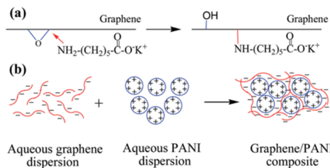
Зураг 6 (a). Усанд дисперс үүсгэх чадвартай графене бэлтгэх болон (b) графене полианалин нэгдэл үүсгэх схемчилсэн загвар
