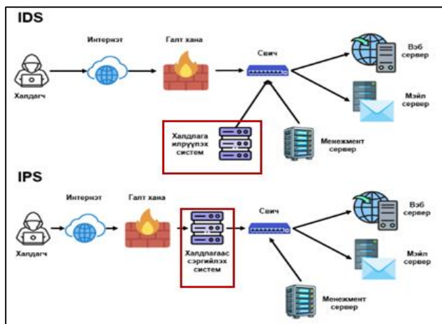
Fig. 1. IDS/IPS-ийн ажиллах зарчим
